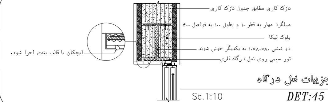
جزئیات فعلی در گاه DET:44 Sc. 1:10
