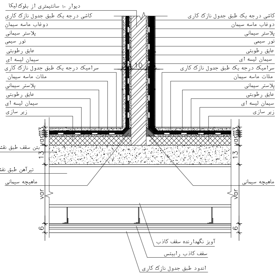
جزئیات دیوار ۱۰ سانتیمتری و نحوه عایق بندی سرویس در طبقه DET:41 Sc. 1:10
