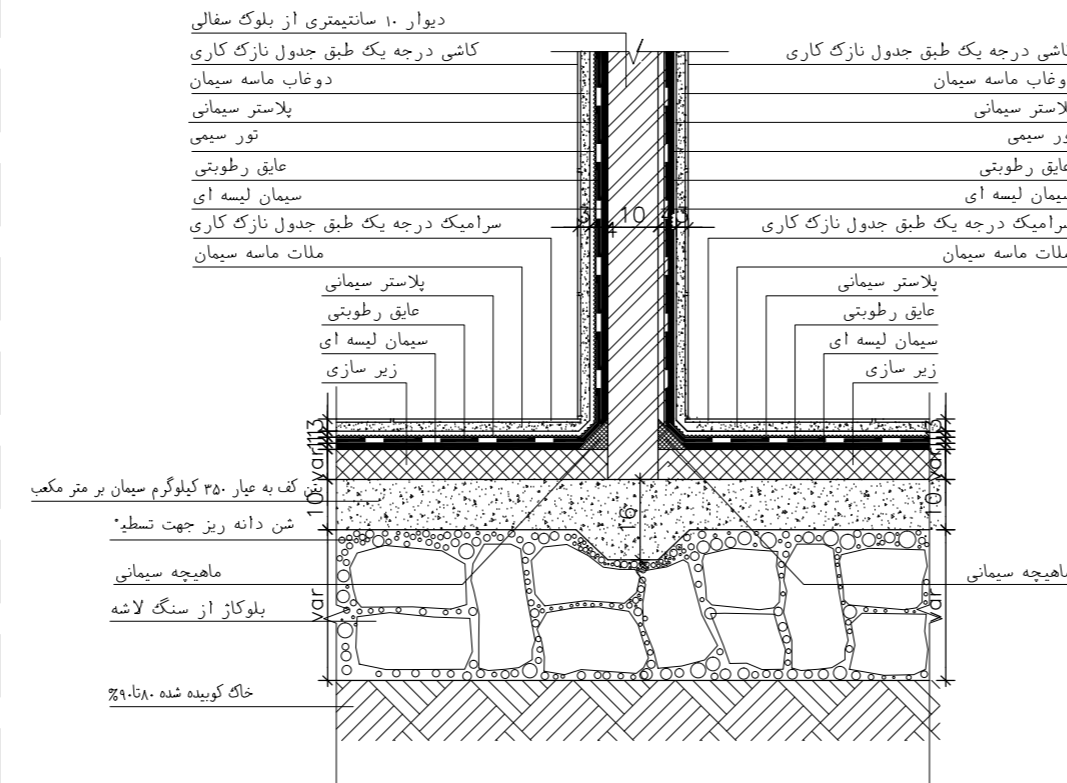
جزئیات دیوار ۱۰ سانتیمتری و نحوه عایق بندی سرویس در همکف DET:42 Sc. 1:10
