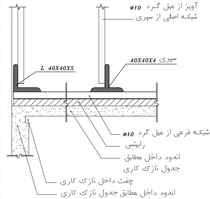
جزئیات اتصال سقف گاذب به دیوار DET:39 SC. 1:10 (کناف پامشابه)
