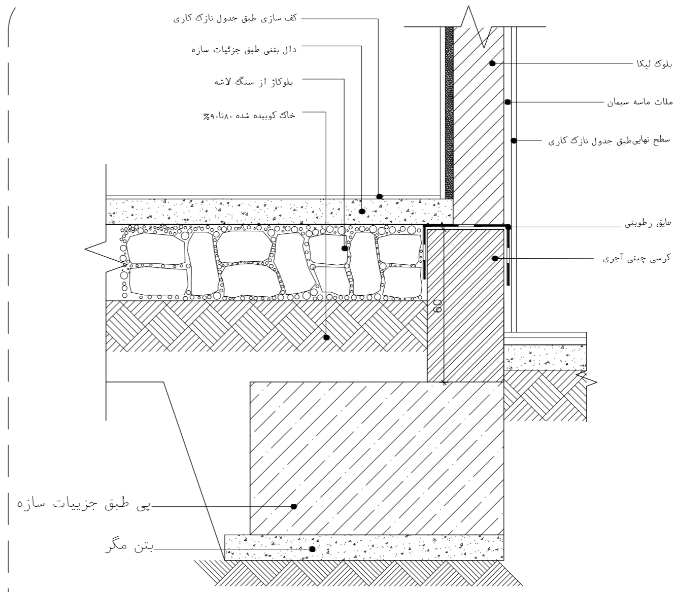
نحوه اجرای دیواره خارجی در همکف DET:43 SC. 1:10
