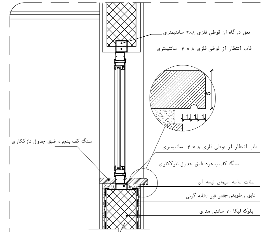
جزئیات اجرایی کف پنجره DET:40 SC. 1:10
