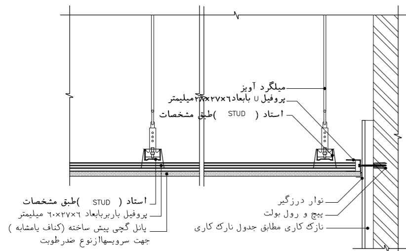
جزئیات سقف گاذب پانل گچی کناف DET:38 SC. 1:10 (کناف پامشابه)
