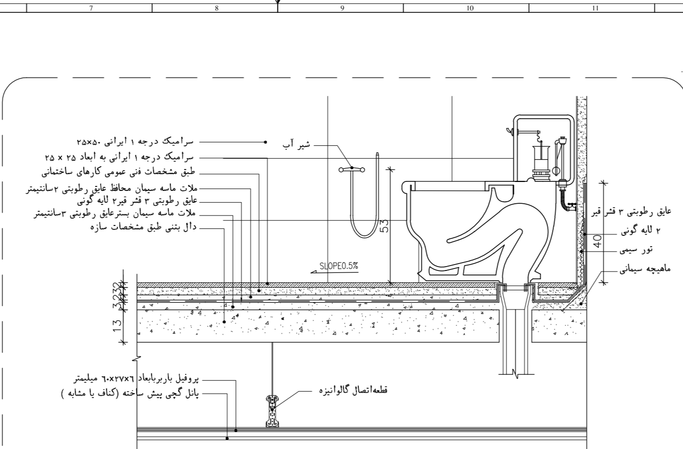
جزئیات اجرایی توالت فرنگی در طبقه DET:34 SC. 1:10
