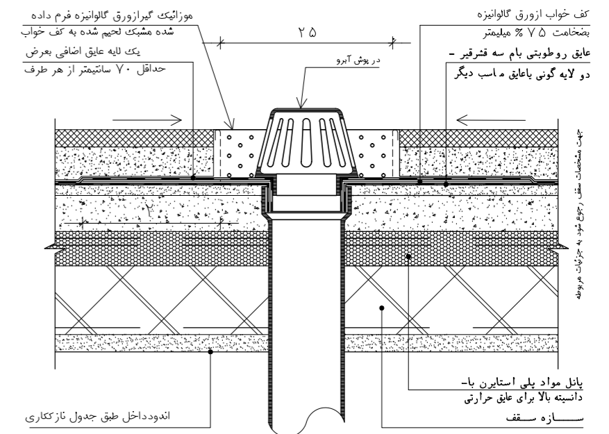
جزئیات کشور آبرو DET:35 SC. 1:5
