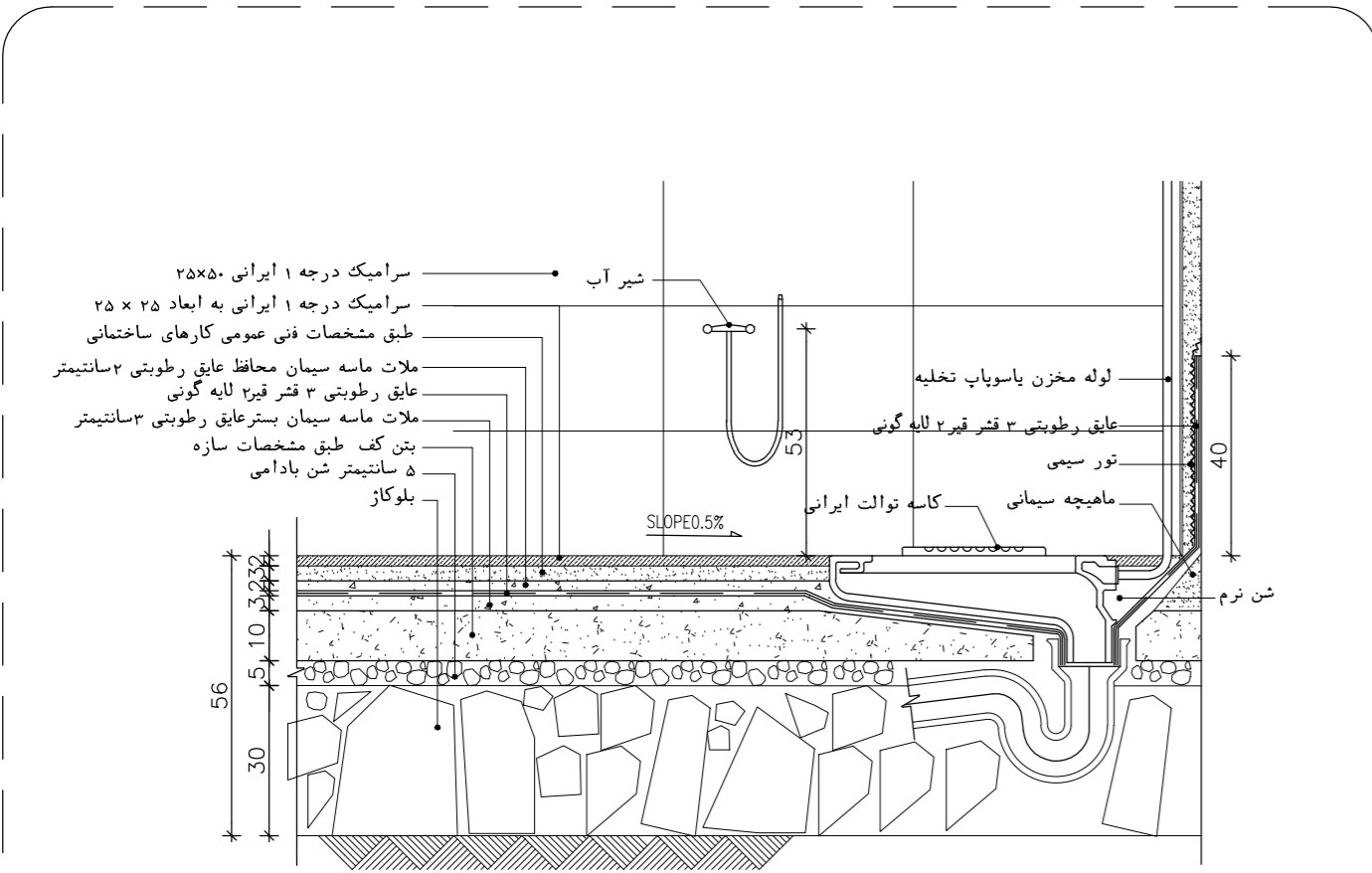
جزئیات اجرایی توالت ایرانی در همکف DET:36 SC. 1:10
