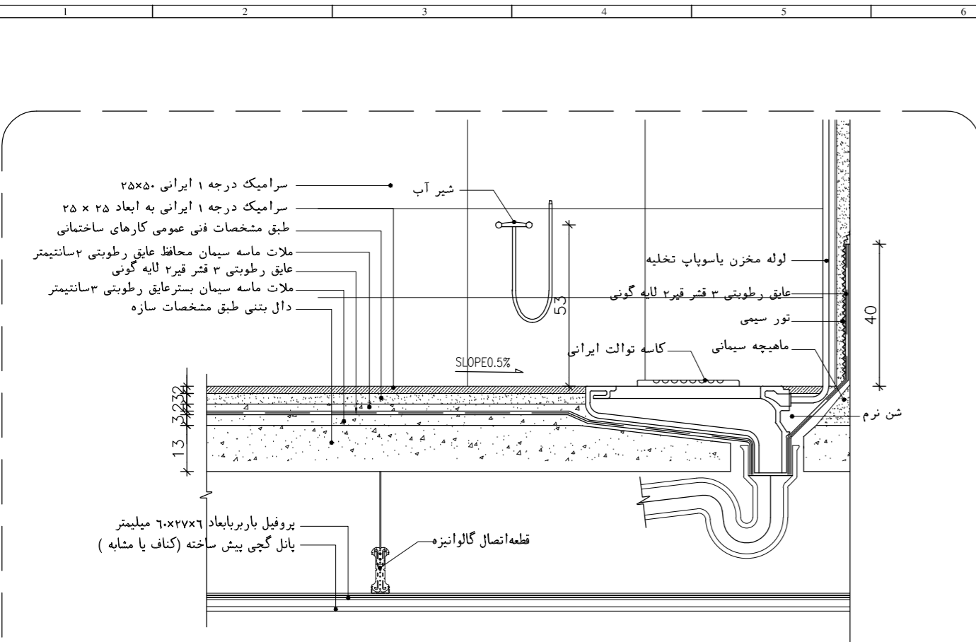
جزئیات اجرایی توالت ایرانی در طبقه DET:33 SC. 1:10
