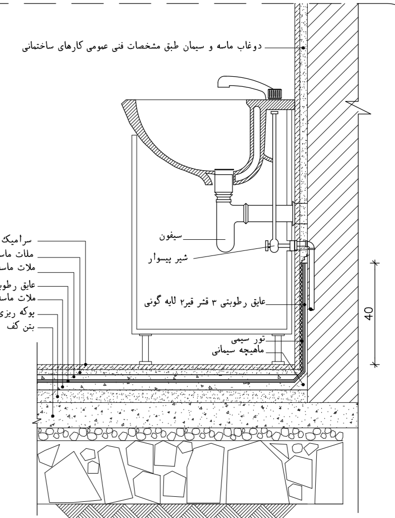
جزئیات دستشویی و اتصالات آن DET:37 SC. 1:10
