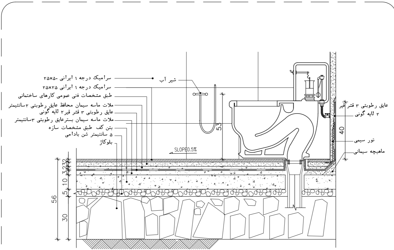
جزئیات اجرایی توالت فرنگی در همکف DET:36 SC. 1:10
