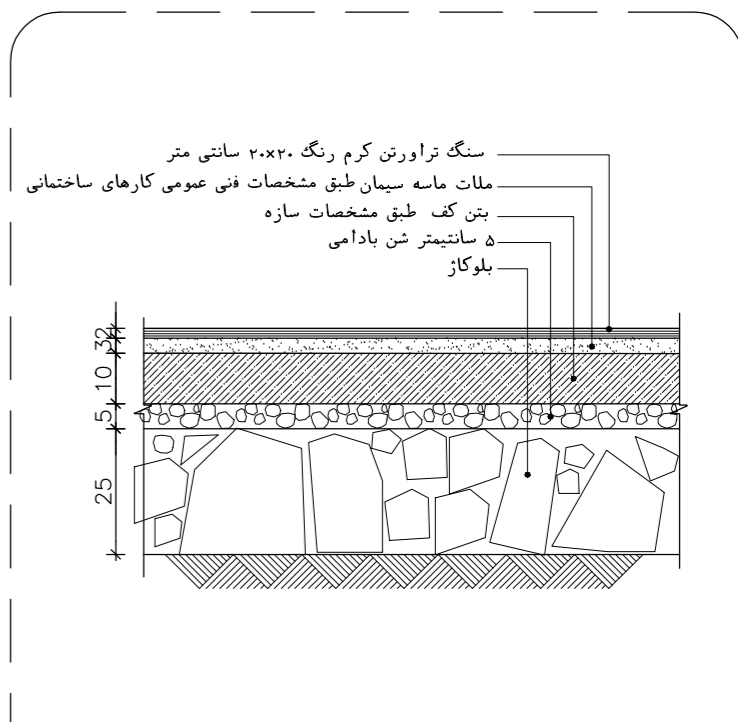
جزئیات کف سازی حیاط SC. 1:10
