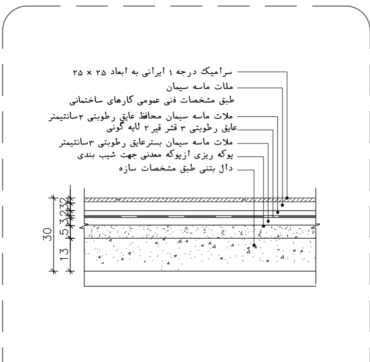
جزئیات کف سازی فضای مرطوب در طبقه SC. 1:10
