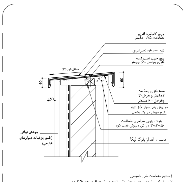
جزئیات اجرایی فلاشینگ با م SC. 1:5
