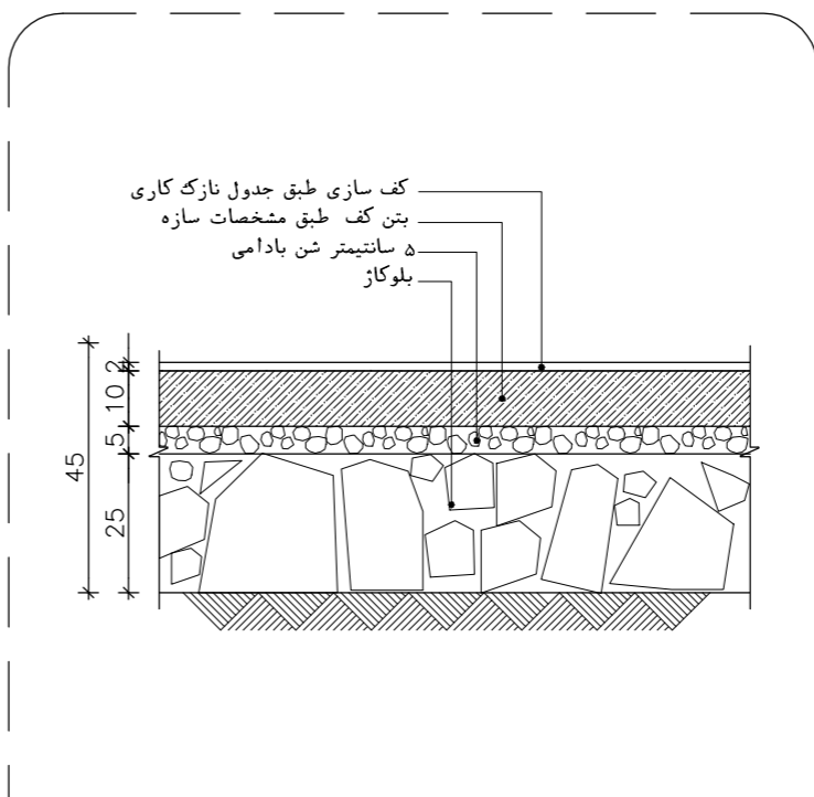
جزئیات کف سازی در همکف SC. 1:10
