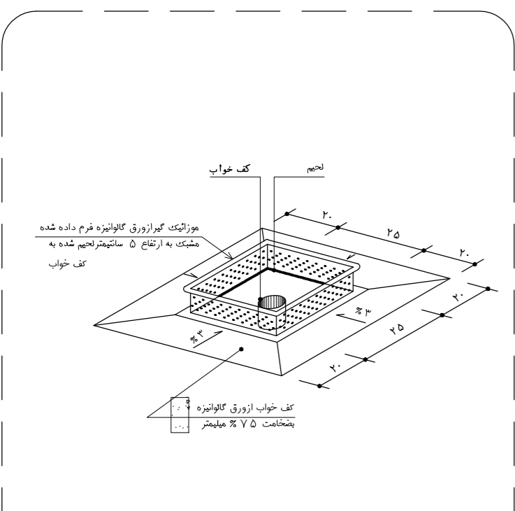
جزئیات کف سازی آشپزخانه SC. 1:10
