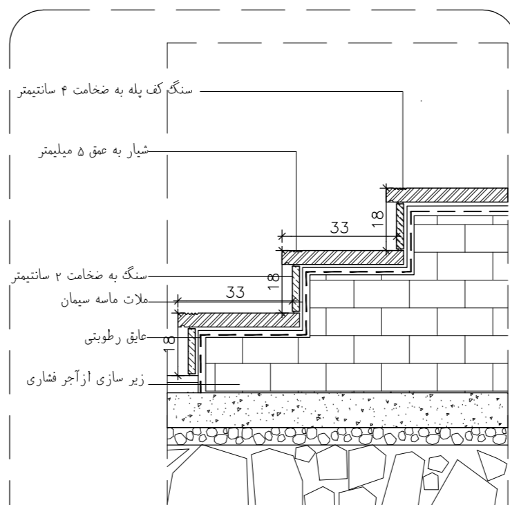
جزئیات اجرایی پله خارجی SC. 1:10
