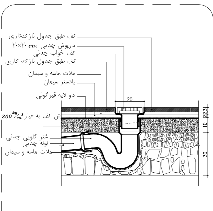
جزئیات کف شویی در همکف SC. 1:10
