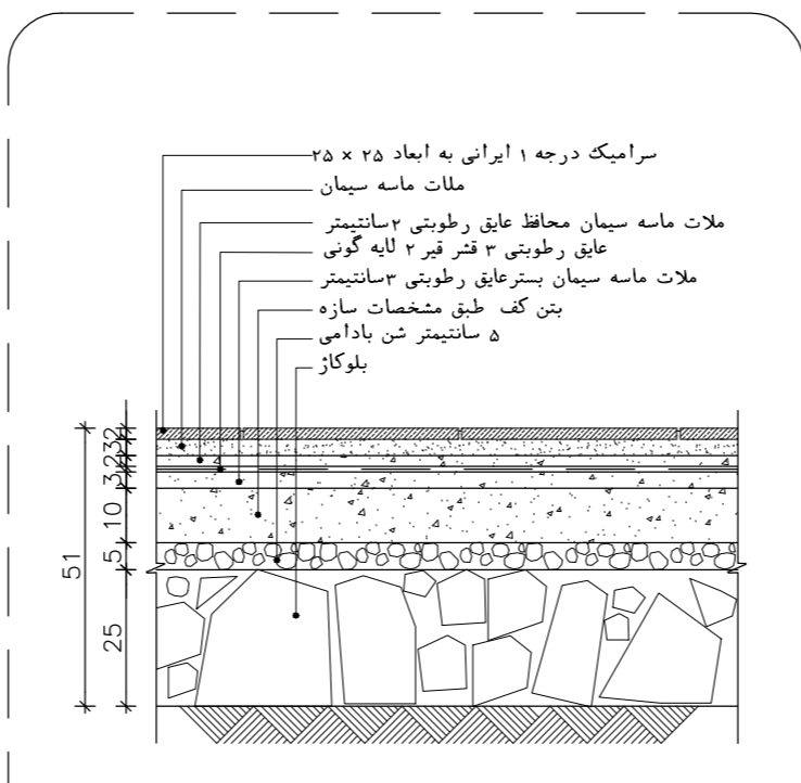
جزئیات کف سازی فضای مرطوب در همکف SC. 1:10
