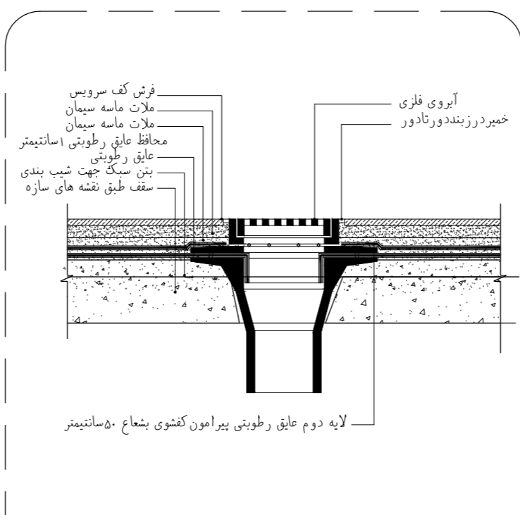
جزئیات اجرایی کف آشپزخانه SC. 1:10
