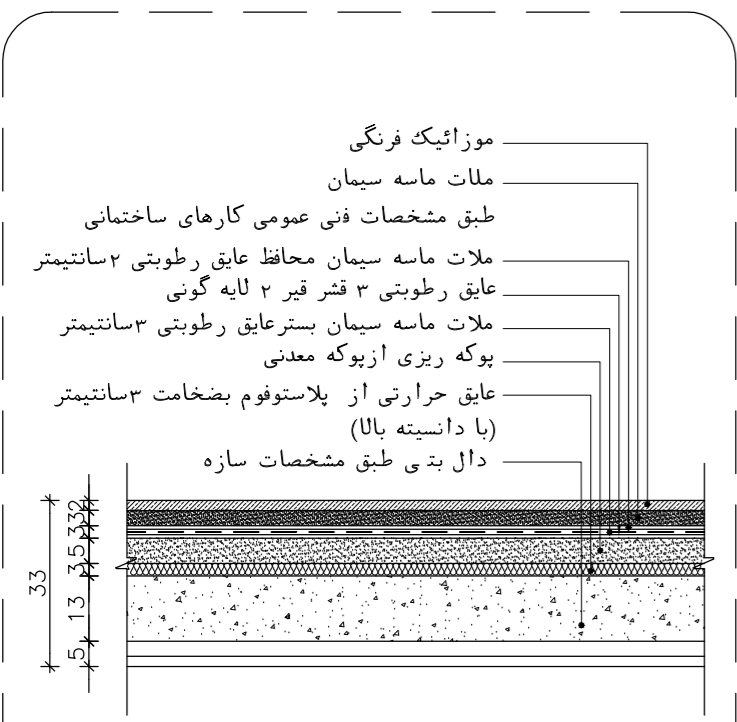
جزئیات کف سازی با موزائیک SC. 1:10
